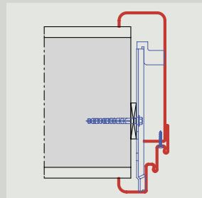
2-részes U-tok, pofaszélesség állítással, duplafalalal és rádiuszokkal Dübeles szerelés
