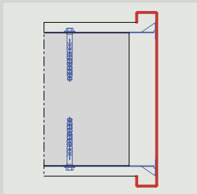
Átjárótok Szerelés kihajtható szerelő lemezzel
