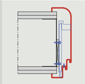
2-részes U-tok, pofaszélesség állítás nélkül és rejtett osztással, duplafalccal és rádiusszal Dűbeles szerelés
