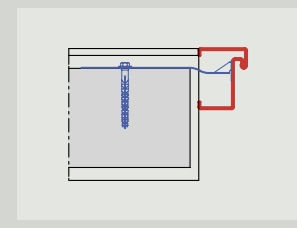
Blokktok, sportcsarnokokhoz Szerelés kihajtható szerelő lemezzel
