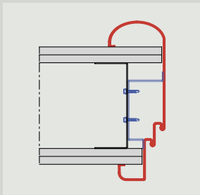
U-tok, kerek alakú, duplafalalal Szerelés kalapprofilal
