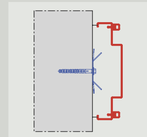
Ablaktok, blokktokként, dupla üvegezéshez Szerelés dübellel
