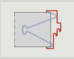
U-tok, gipszfallóhoz, duplafalalal és diszfalalal Szerelés drótkampóval
