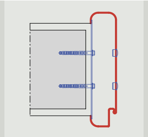
U-tok, rádiuszokkal Szerelés dűbelezéssel
