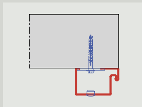
Keret-tok, a fal elé való beépítéshez Szerelés dűbelezéssel
