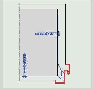
Saroktok Szerelés kihajtható szerelő lemezzel
