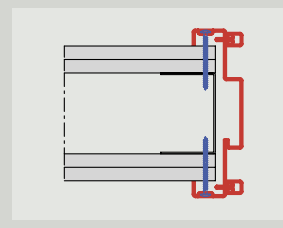
2-részes ablaktok, dupla üvegezéshez Szerelés szerelő lyukakon toktükrön keresztül
