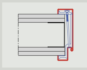
U-tok, utólagos beépítéshez Szerelés aluminium szorítópórákkal, rejtett szerelés
