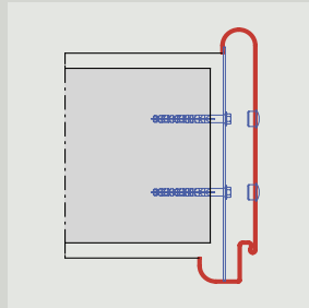
U-tok, rádiuszokkal Szerelés dübelezéssel
