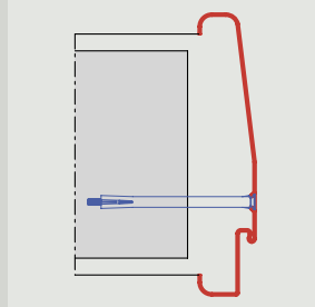
U-tok, ferde kávéval és rádiuszokkal Típlis szerelés a kávéban elhelyezett Tütung-lyukon keresztül
