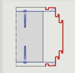
Dupla ajtók, ellenoldali nyitási irányhoz, duplafalalal és árnyékhorronnyal Szerelés kihajtható szerelő lemezzel
