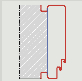
U-tok, betonfalakhoz, duplafalalal, árnyékhorronnyal és rádiuszokkal Szerelés laposvassal, betonkiöntéses eljárással
