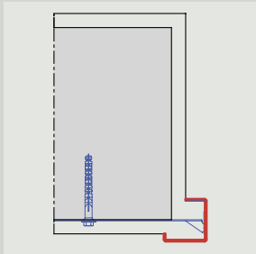
Ellentok, élvédőként Szerelés kihajtható szerelő lemezzel
