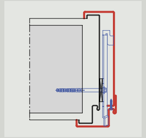
Kétrészes U-tok, pofaszélesség-állítással, meglévő tok fölé való beépítéshez Szerelés dűbeles szereléssel
