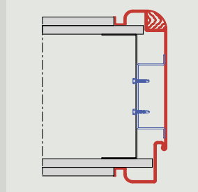
U-tok, kórházakhoz; ütközőélel, árnyékhorronnyal és rádiuszokkal Szerelés kalapprofilal
