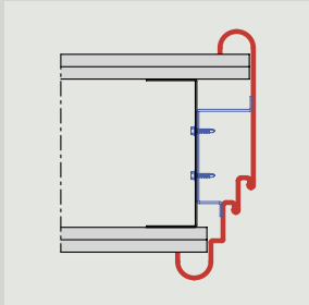
U-tok ujjbecsípődésvédelemmel és duplafalalal Szerelés kalapprofilal
