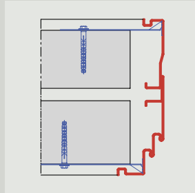
Dilatációs fuga-tok, duplafalalal és árnyékhorronnyal Szerelés kihajtható szerelő lemezzel
