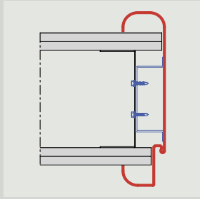
U-tok, rádiuszokkal Szerelés kalapprofilal
