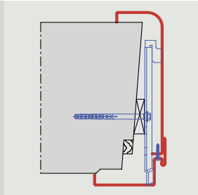
2-részes U-tok, pofaszélesség állítás és rádiusszal Dűbeles szerelés
