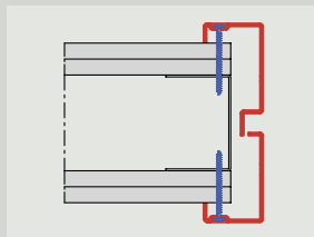
Ablaktok, közepén lévő üvegezéshez Szerelés a toktükrőben szerelő lyukakon
