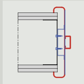
Lengőajtók, rádiuszokkal Szerelés kalapprofilal
