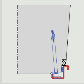
Szanáló saroktok Dűbeles szereléssel
