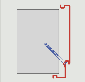
U-tok, árnyékhorronnyal Dűbeles szerelés gumitömítés alatt
