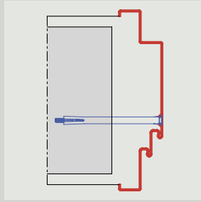
U-tok, duplafalccal és díszfalccal Dűbeles szereléssel
