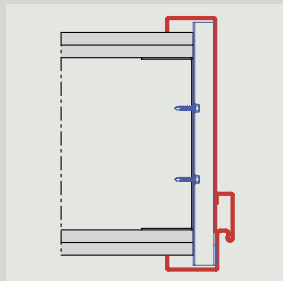
2-részes U-tok, pofaszélesség állításal Dűbeles szerelés
