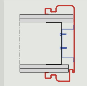
U-tok, különleges profil alakú Szerelés kalapprofilal
