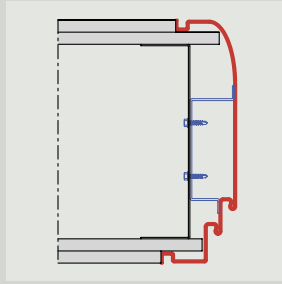
U-tok, ívelt alakú, duplafalccal és árnyékhorronnyal Szerelés kalapprofilal
