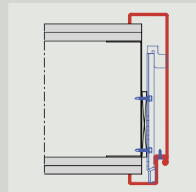
2-részes U-tok, pofaszélesség állítás nélkül és rejtett osztással Dübeles szerelés
