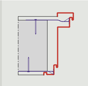
Dupla ajtótok egyoldalas nyitási irányhoz, egyoldali árnyékhorronnyal Szerelés kihajtható szerelő lemezzel
