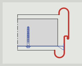
U-tok, ujjbecsípődésvédelemmel Szerelés kihajtható szerelő lemezzel
