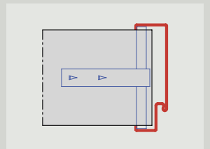
U-tok, gipszfalhoz, szimmetrikus toktükrővel Szerelés tolóhorronnyal
