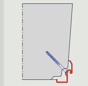
Saroktok profil, szanáláshoz Dübeles szerelés gumitömítés alatt
