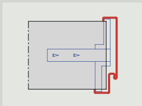
U-tok, gipszfalhoz Szerelés tolóhorronnyal
