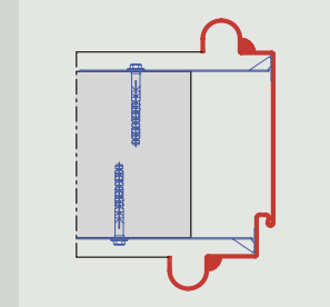
U-tok, különleges profil-alakú Szerelés kihajtható szerelő lemezzel
